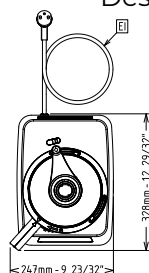
Dessus
